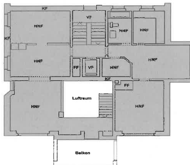
Grundriss 1. Obergeschoss:
