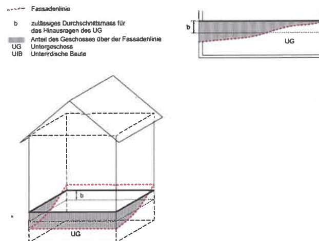
Figur Untergeschosse
